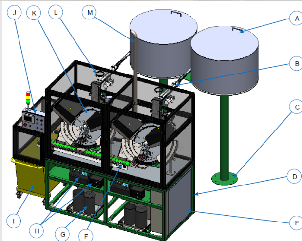
Figur 1 - Overordnet layout
